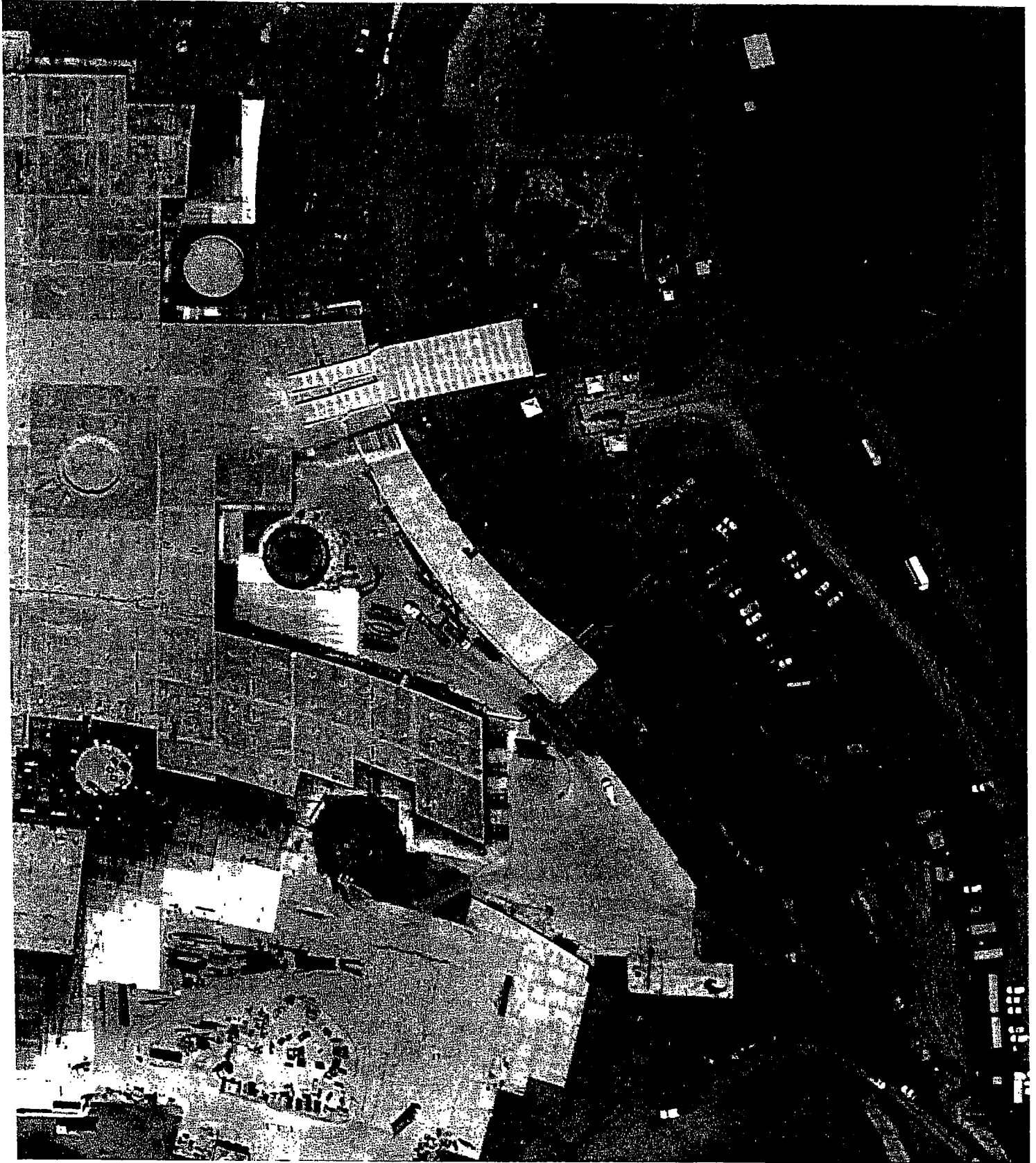
Avance de loza de cimentación del Edificio Terminal, NAIM.
