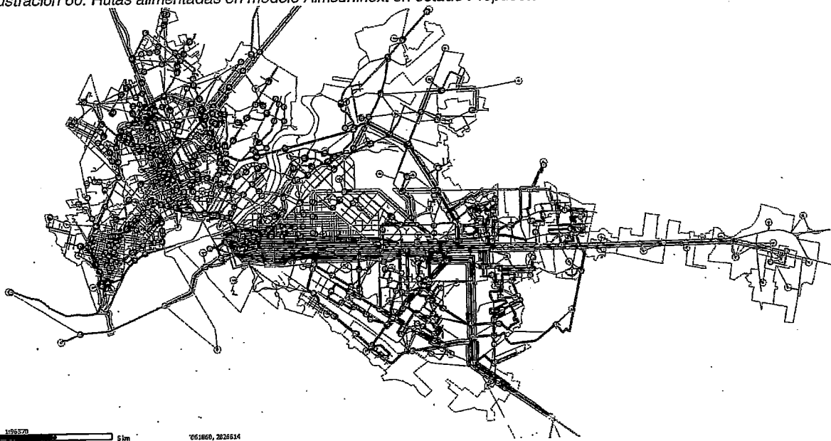
Ilustración 60. Rutas alimentadas en modelo Aimsun.next en estado Propuesto - Coahuila
