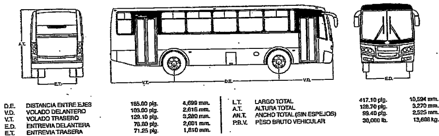
Fuente: Autobuses Mercedes Benz
