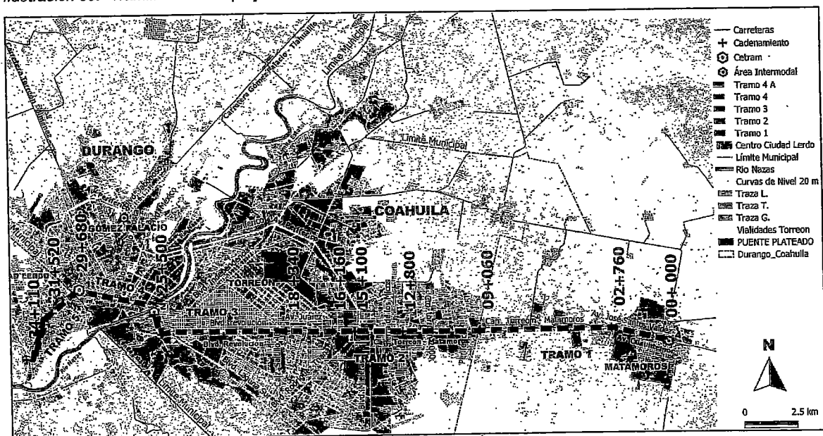
Ilustración 65.- Tramificación del proyecto
