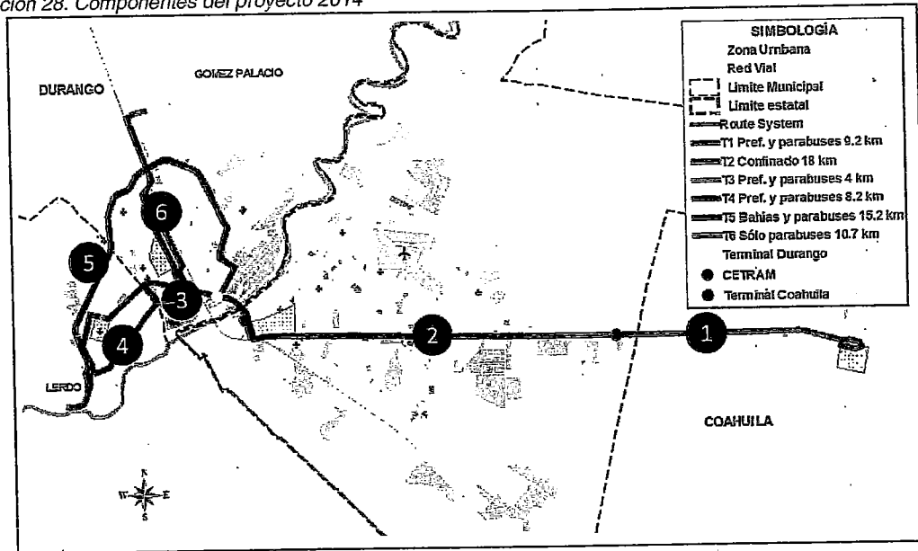
Ilustración 28. Componentes del proyecto 2014
