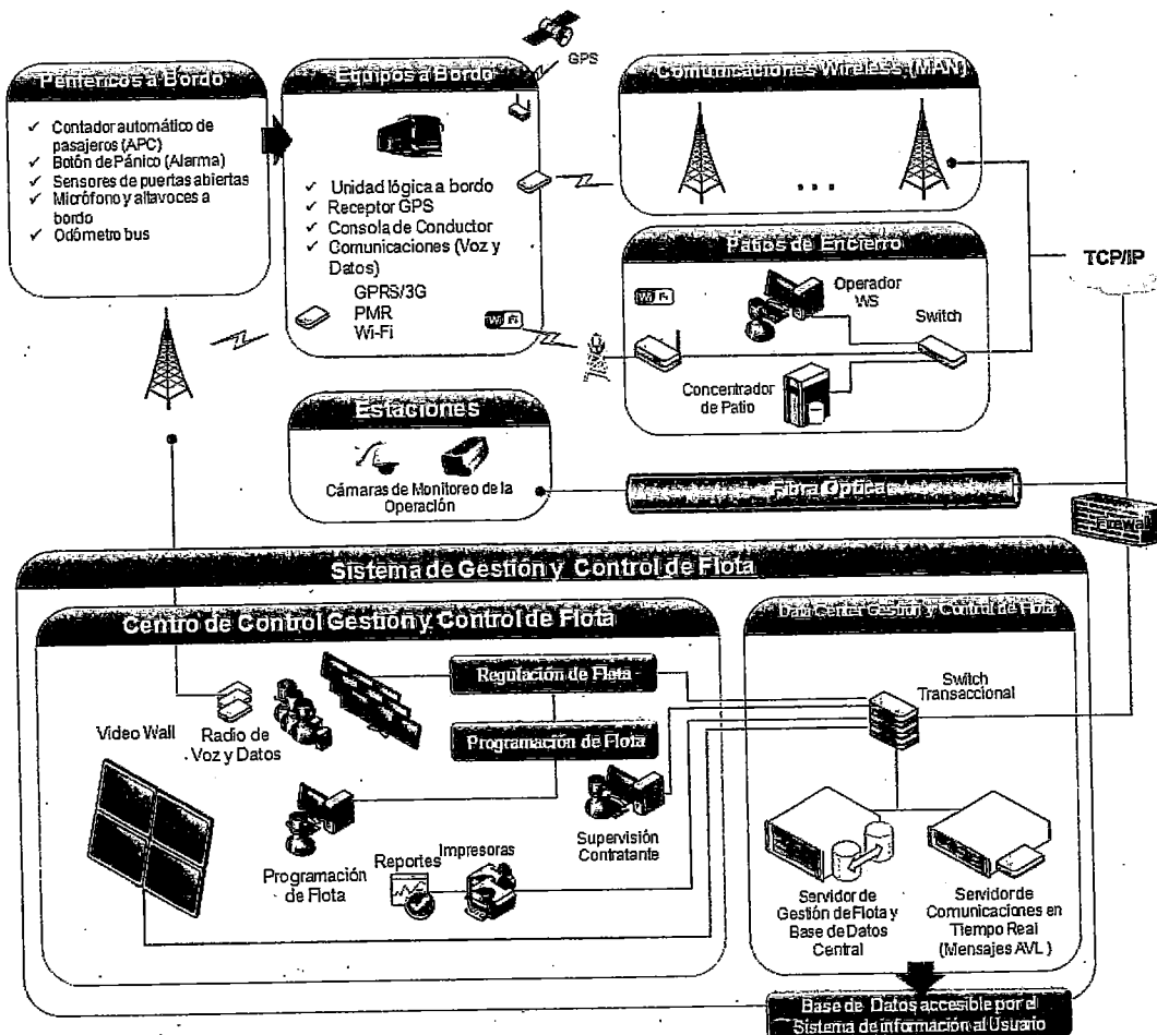
Figura 1. Arquitectura del Sistema de Control de Flota
